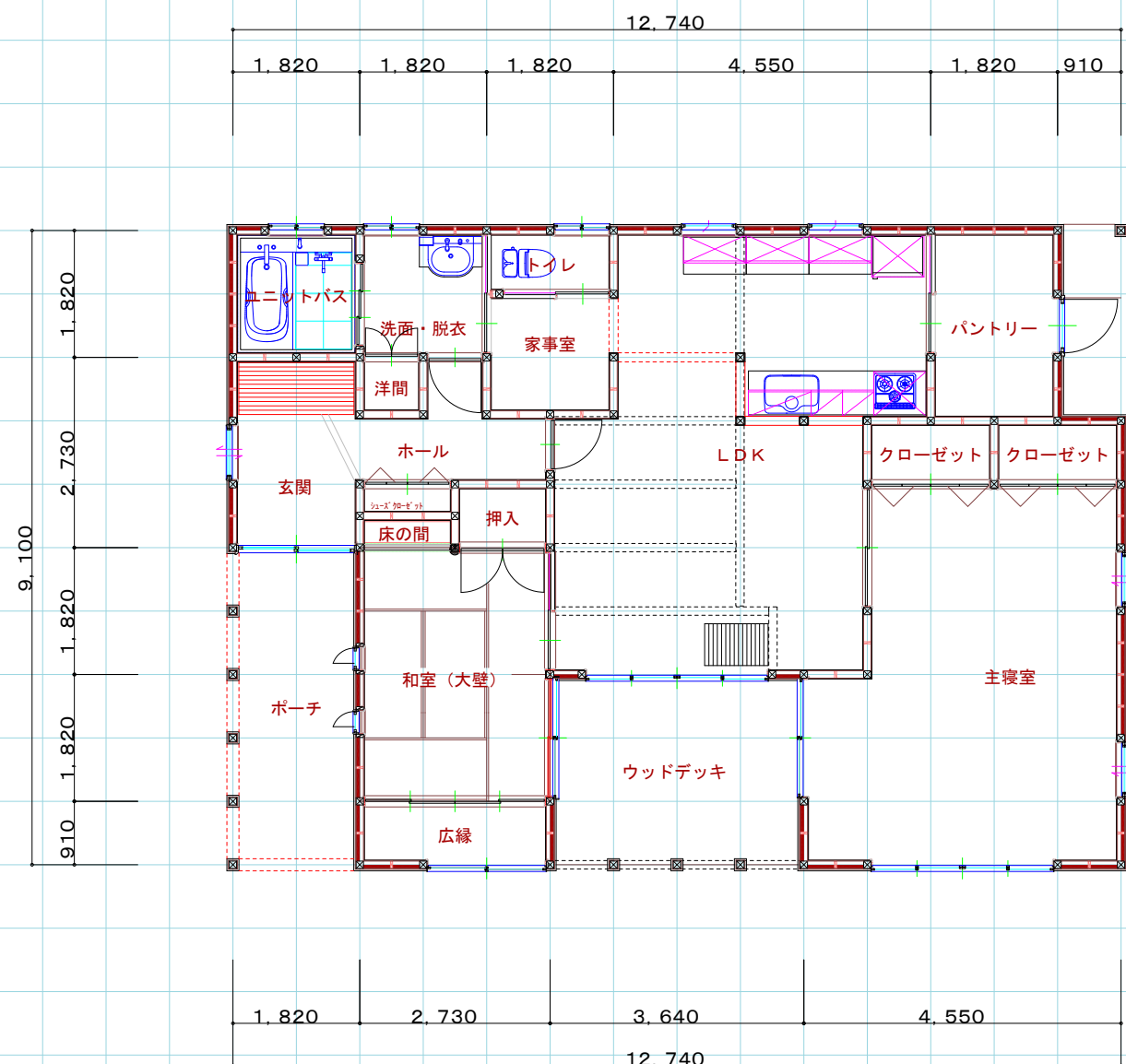
1階平面図
